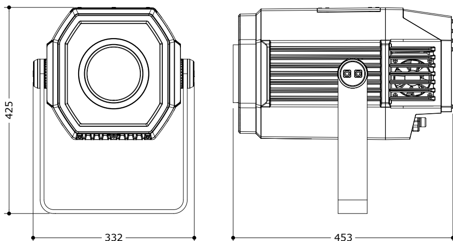
Disegno tecnico
