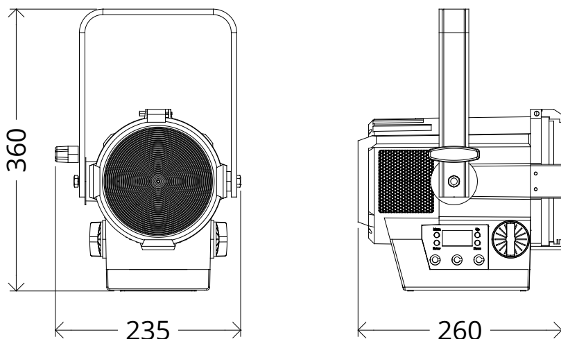
Fig.1 - Disegno tecnico
